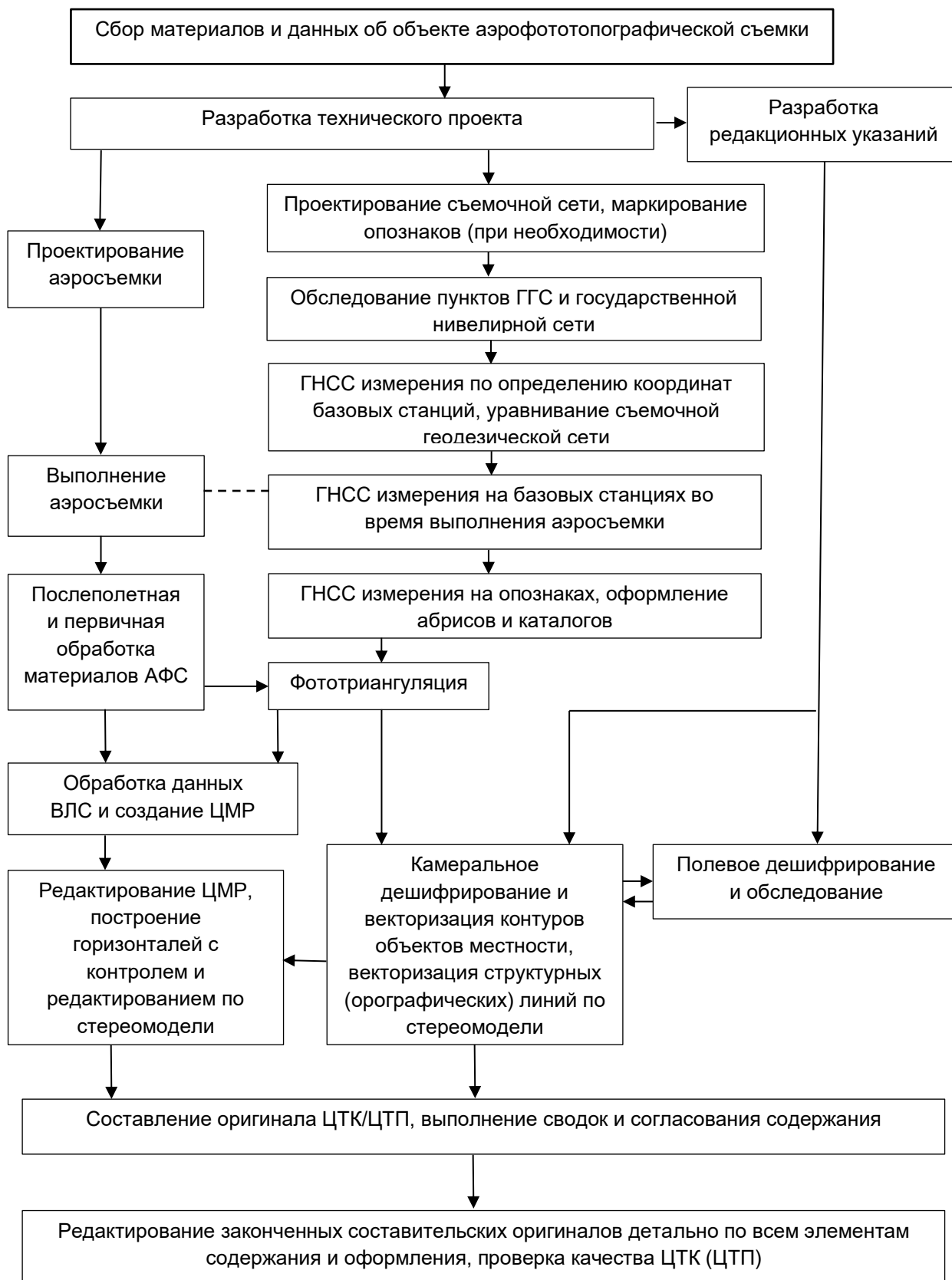
Рисунок А.2–Технологическая схема комбинированной стереотопографической съемки
