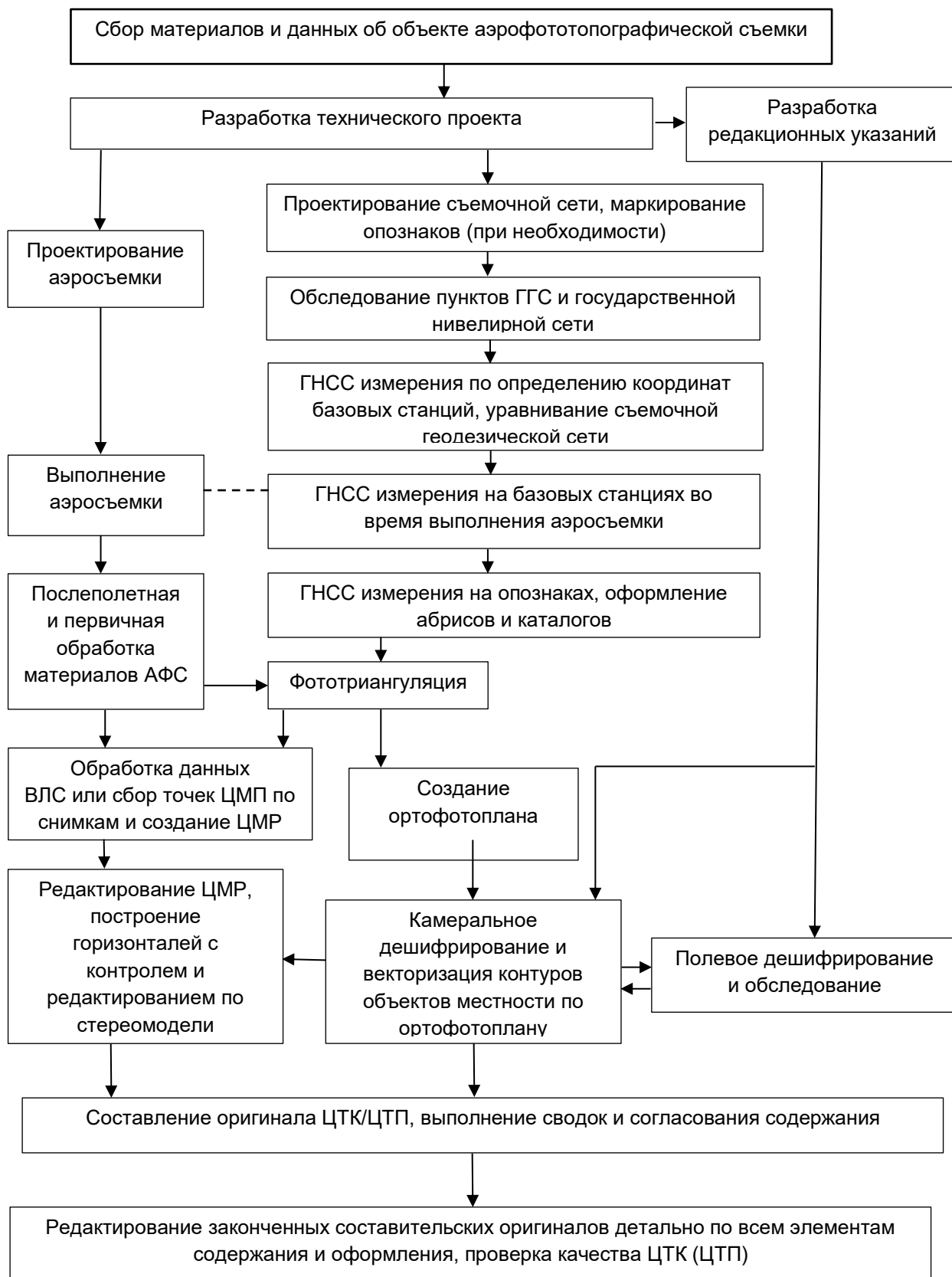
Рисунок А.3 – Технологическая схема комбинированной аэрофототопографической съемки
