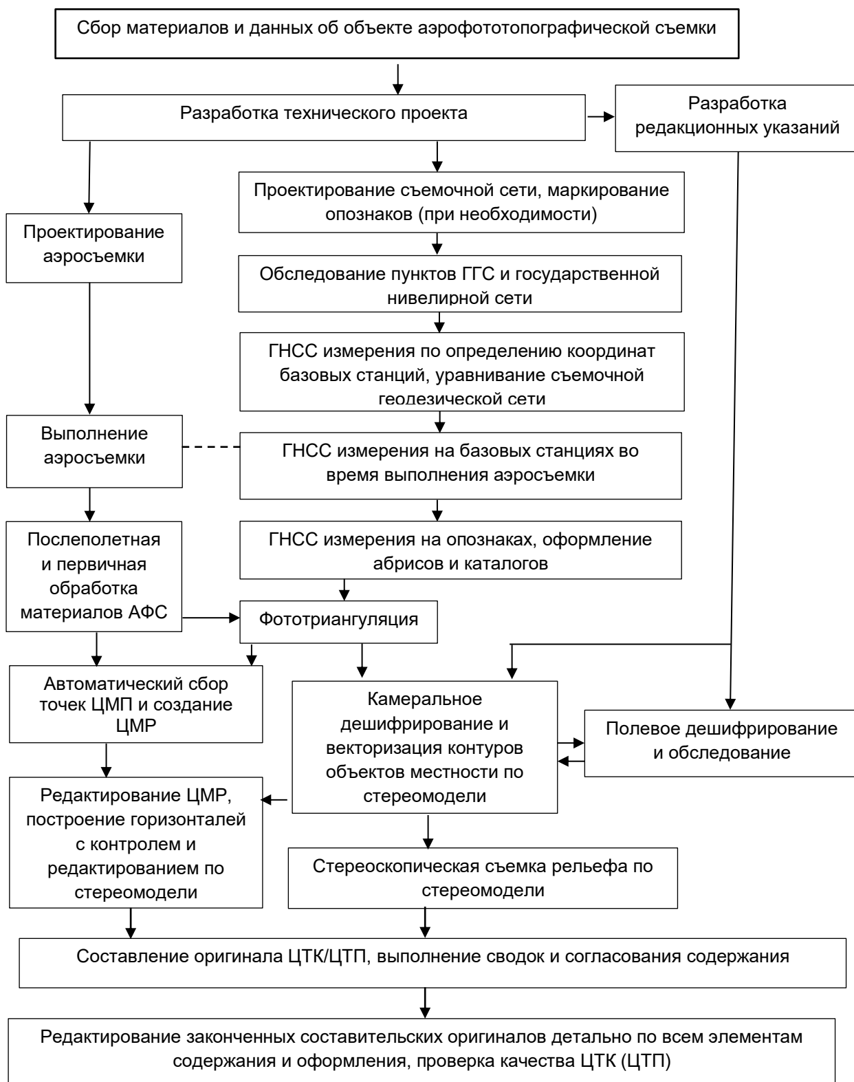
Рисунок А.1—Технологическая схема стереотопографической съемки
